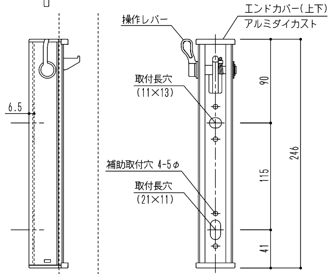
取付ブラケット詳細図
